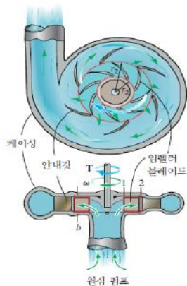
그림 3-14. 원심펌프 구조
